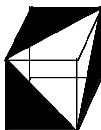
QUARK : tétraèdre vide, trou en creux dans un cube plein
