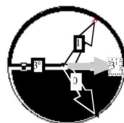
Structure trinaire du Méta-Univers Figure 37
