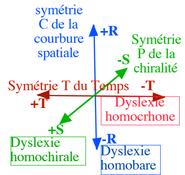
Intrication de l'Interaction à l'échelle quantique Figure 31
