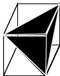
LEPTON : tétraèdre plein, noeud saillant dans le cube vide
